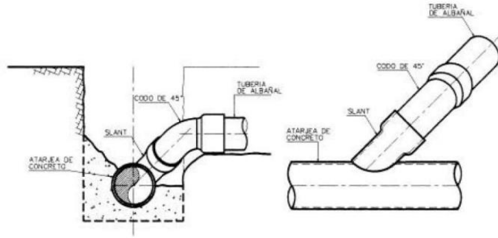
IMG 7. CONEXIÓN A RED DOMICILIARIA.
