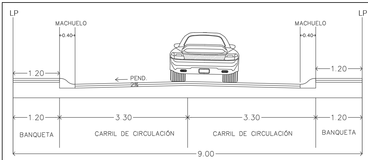
Imagen V-1.- Sección vial en vialidades locales tipo "A"
