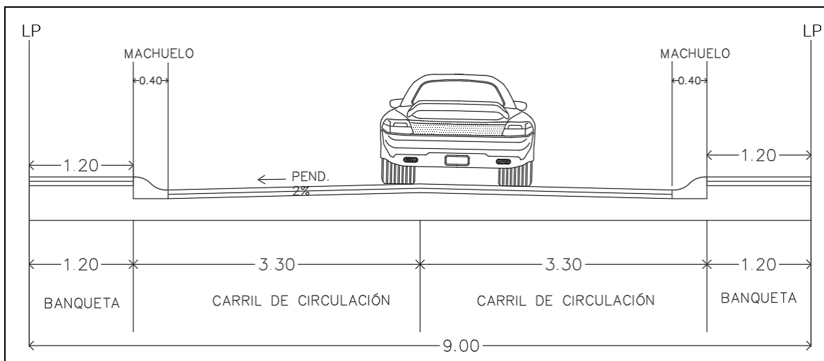
Imagen V-2.- Sección vial en vialidades colectoras tipo "B"
